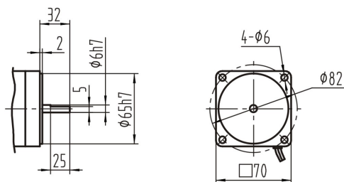
70型脚架
