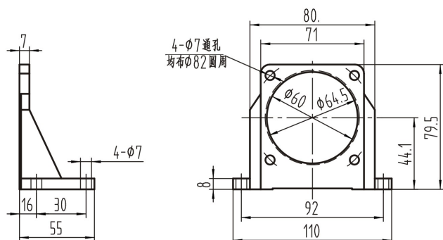
70型脚架
