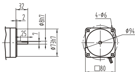
80型脚架
