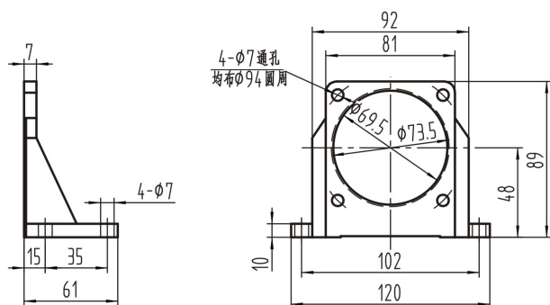
80型脚架
