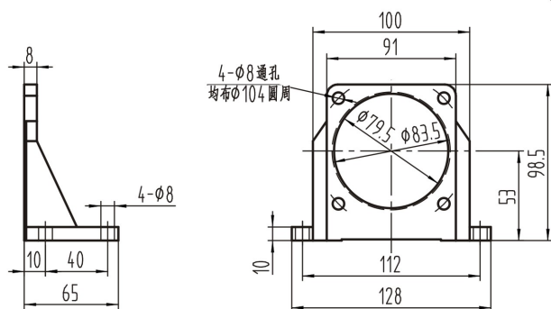
90型脚架
